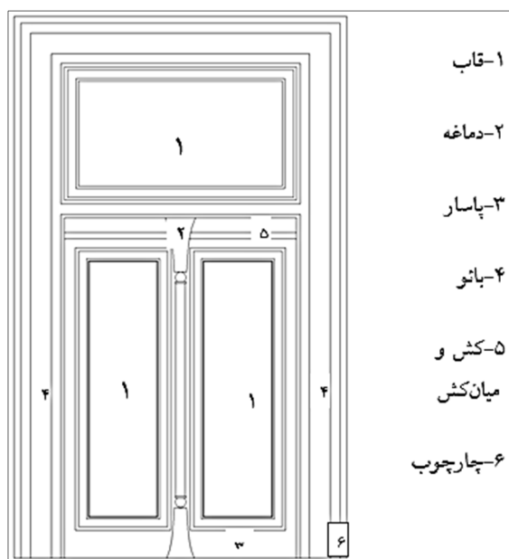
تصویر ۱: اجزای اصلی در، در دوره صفوی Image. 1: Main Components in Safavid Period
