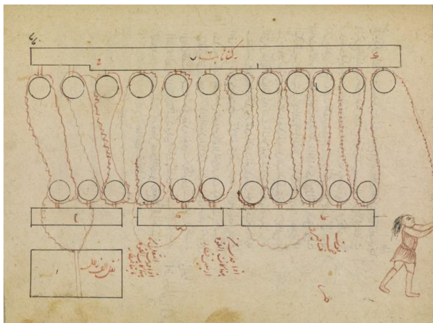
شکل ۱۲. جرثقیل، کتاب فی رفع الأشياء الثقيلة از الإسكندرانی، سده یازدهم/هفدهم، کتابخانه بریتانیا (Add MS 23390، گ 31پ)، (Qatar Digital Library, n.d)
