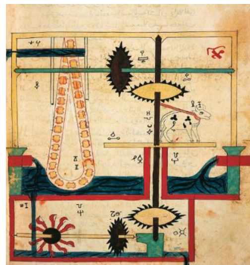
شکل ۱۳. ماشین آبکشی، کتاب الجامع بین العلم و العمل النافع فی صناعة الحیل، جزری، سده هفتم/سیزدهم، کتابخانه کاخ توپقاپی (MS Ahmet III 3472، گ 154پ).
