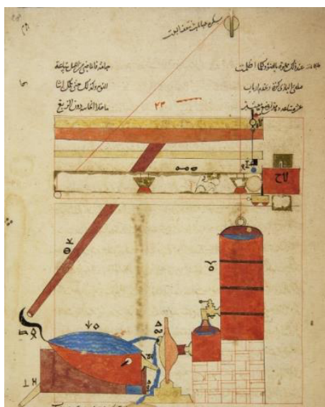
شکل ۴. ساعت آبی فواره‌دار، کتاب الجامع بین العلم و العمل النافع فی صناعة الحیل، بدیع‌الزمان الجزری، سده یازدهم/هفدهم، کتابخانه دولتی برلین (Or. Fol. 3306، گ 23)، (publicdomainreview, n.d).
