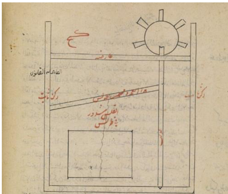
شکل ۱۱. دستگاه بالابر، کتاب فی رفع الأشياء الثقيلة از الإسكندرانی، سده یازدهم/هفدهم، کتابخانه بریتانیا (Add MS 23390، گ 21پ)، (Qatar Digital Library, n.d)
