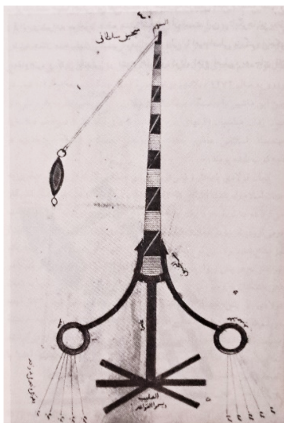
شکل ۸. نوعی منجنیق کششی، سده هشتم/چهاردهم، کتابخانه کاخ توپقاپی (حسن و هیل، ۱۳۷۵، ص. ۱۳۷).
