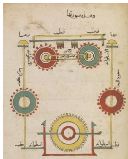
شکل ۱۵. دستگاهی برای استخراج آب از چاه، کتاب الحیل فی الحروب و فتح المدائن و حفظ الدروب، ابن منکلی، قرن دهم یا یازدهم هـ.ق، کتابخانه بریتانیا (Add MS 14055، گ 160).
