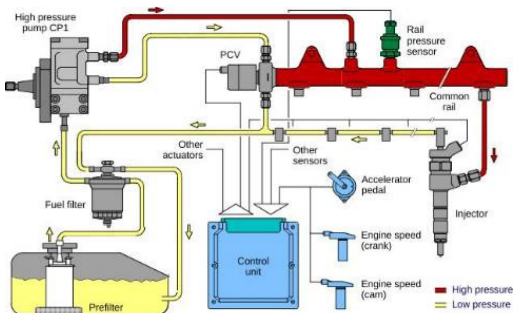
شکل ۱۷. اینفوگرافیک به روش نمودار شماتیک، سیستم تزریق سوخت دیزل با شیر کنترل فشار (dieselnet, n.d).
